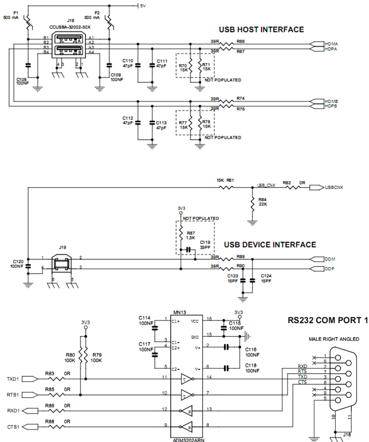
Hình 5.18 Giao tiếp USB và RS232
