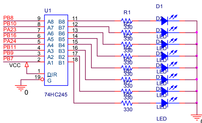
Hình 4-3- Sơ đồ kết nối 8 LEDs đơn.
