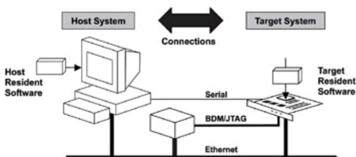
Hình 1-1 Kết nối trong quá trình phát triển hệ thống nhúng
