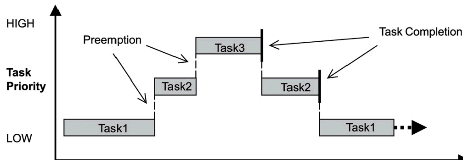
Hình 1-6 Giải thuật lập lịch Preemptive Priority-Based scheduling
